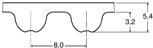
Тип 8М (номинальный размер в мм)
